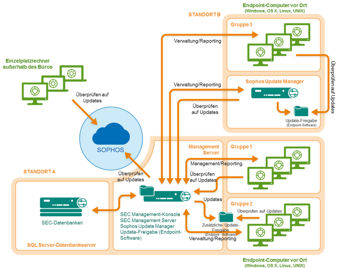
Abbildung 2: Beispiel eines Einsatzszenarios: Zusätzlicher Update Manager, der vom primären Update Manager seine Updates bezieht.
