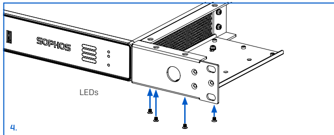
6a. Rackmontage
